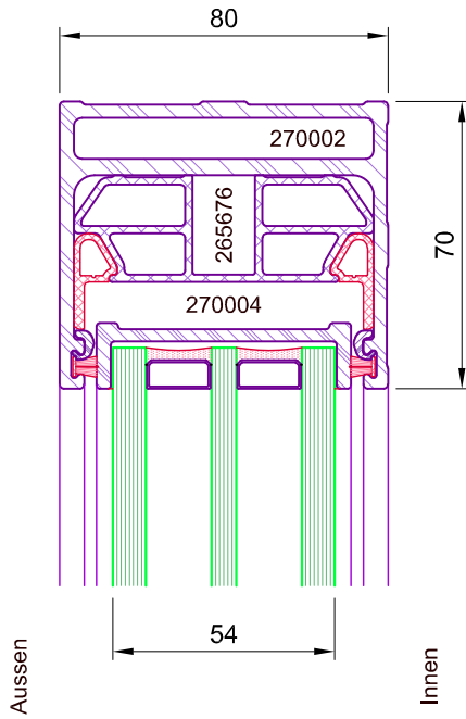
Schnitt durch Schiebeflügel
