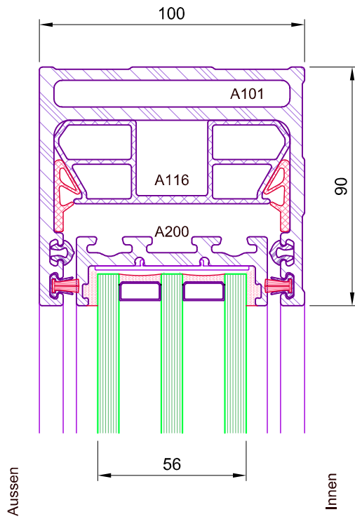
Schnitt durch Schiebeflügel
